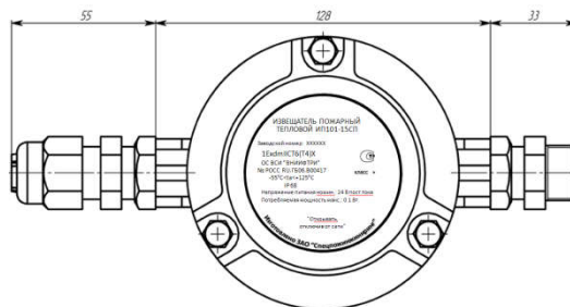
Рисунок 1 – Внешний вид извещателя
