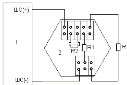
Рисунок 2. Схема подключения извещателя к пультам, использующим импульсы постоянного тока одной полярности или постоянный ток.
