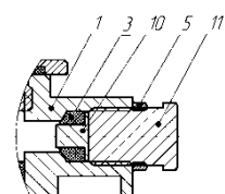
в) монтаж заглушки
