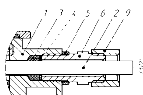
б) монтаж в трубной разводке или металлорукавом
