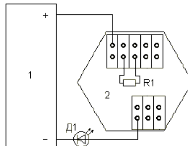
Рисунок 4. Схема подключения извещателя для проверки температуры срабатывания нормально разомкнутого ключа.
