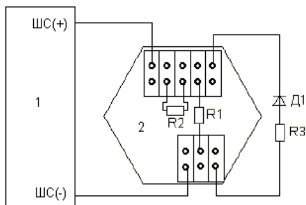
Рисунок 1. Схема подключения извещателя к пультам, использующим импульсы разной полярности
