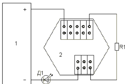
Рисунок 3. Схема подключения извещателя для проверки температуры срабатывания нормально замкнутого ключа.
