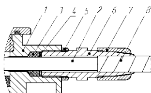
а) монтаж бронированным кабелем
