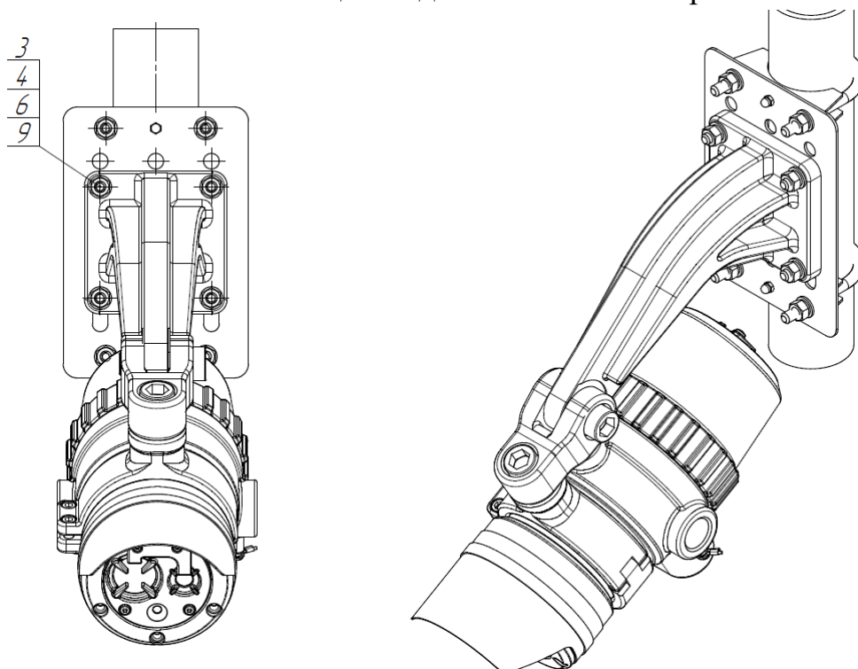
Рис.2 – Изображение установки извещателя пламени «СПАРК»
