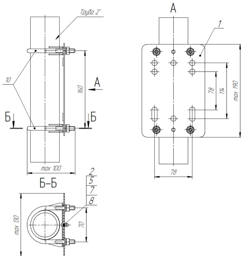
Рис.1 – Общий вид монтажного набора
