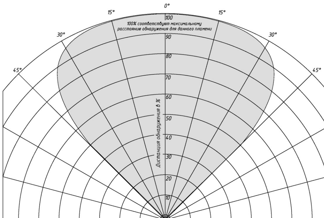
Рисунок 4 — Диаграмма угла обзора извещателя
