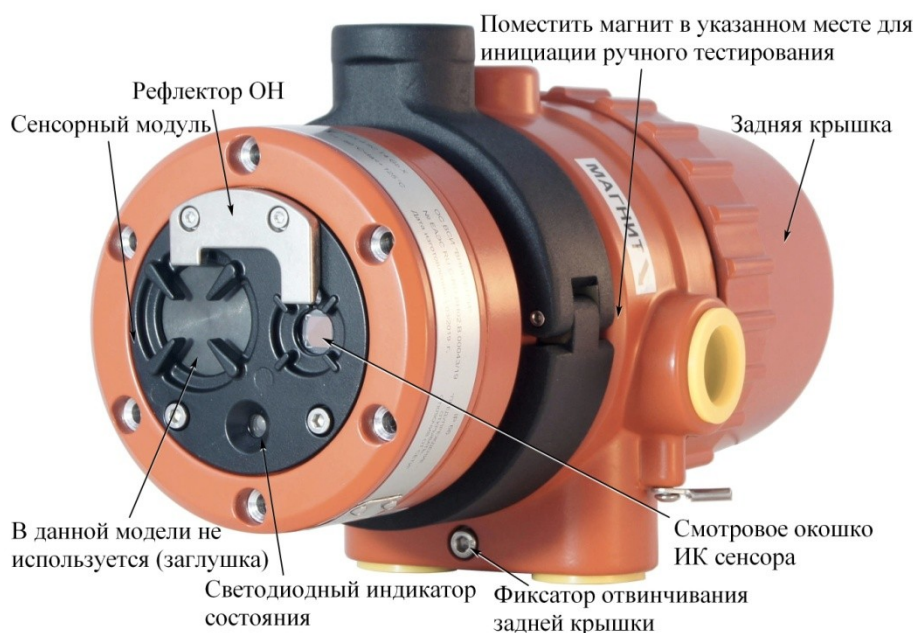
Рисунок 1 – Общий вид извещателя «СПАРК» ИП 330/1-20
