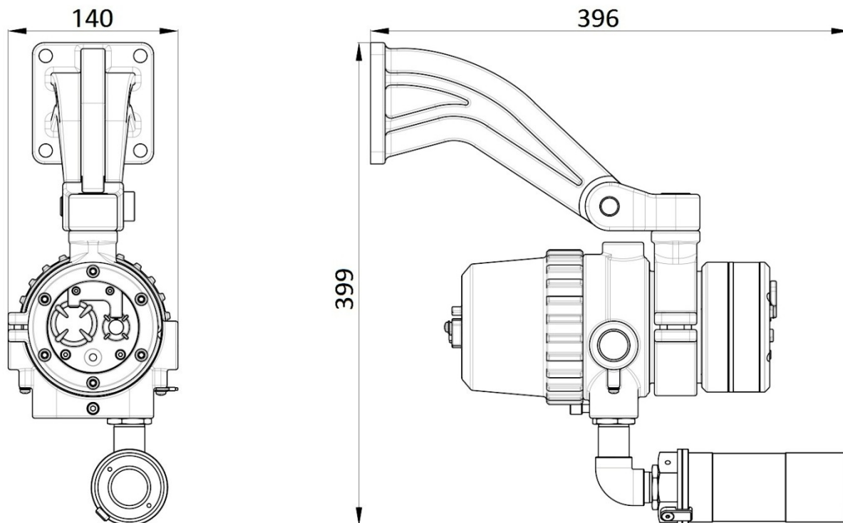
Рисунок 7а– Габаритные размеры извещателя «СПАРК» ИП 330/1-20 с видеокамерой, кронштейном монтажным извещателей пламени «СПАРК» и хомутом монтажным «СПАРК»
