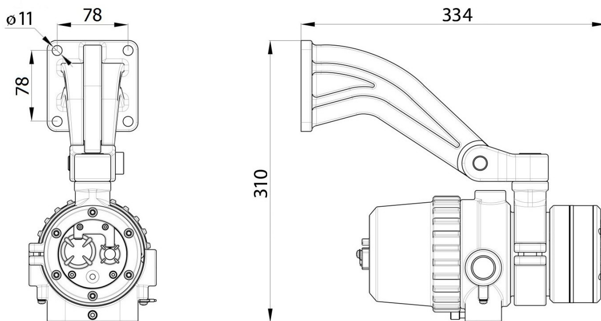
Рисунок 7 – Габаритные размеры извещателя «СПАРК» ИП 330/1-20 с кронштейном монтажным извещателей пламени «СПАРК» и хомутом монтажным «СПАРК»
